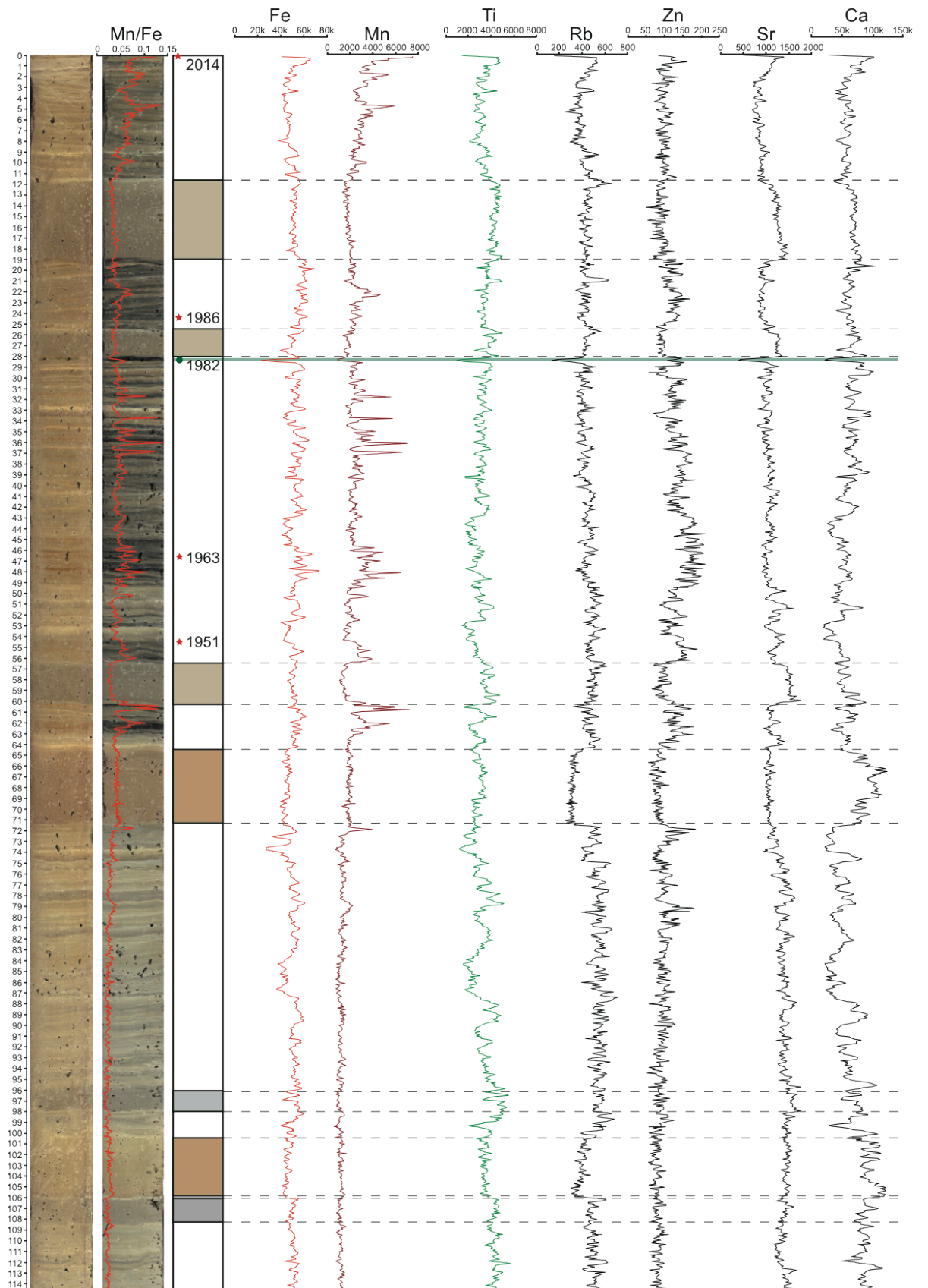
Abbildung 4. XRF signal (counts) im Kern ZUR-LAC-14-01
