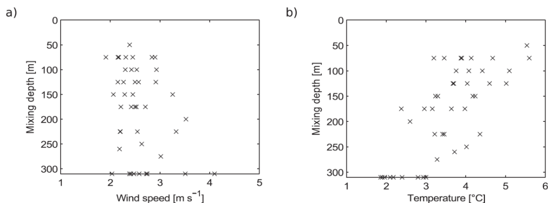
Figur A3: Die Beobachtung, dass die maximale Mischungstiefe kaum vom Wind im Winter abhängt, zeigte sich nicht nur im Zugersee, sondern auch im Genfersee. In der Figur ist die Abhängigkeit der maximalen Mischungstiefe im Genfersee von der Lufttemperatur für die Winter von 1970 bis 2012 dargestellt (aus Schwefel et al. 2016).
