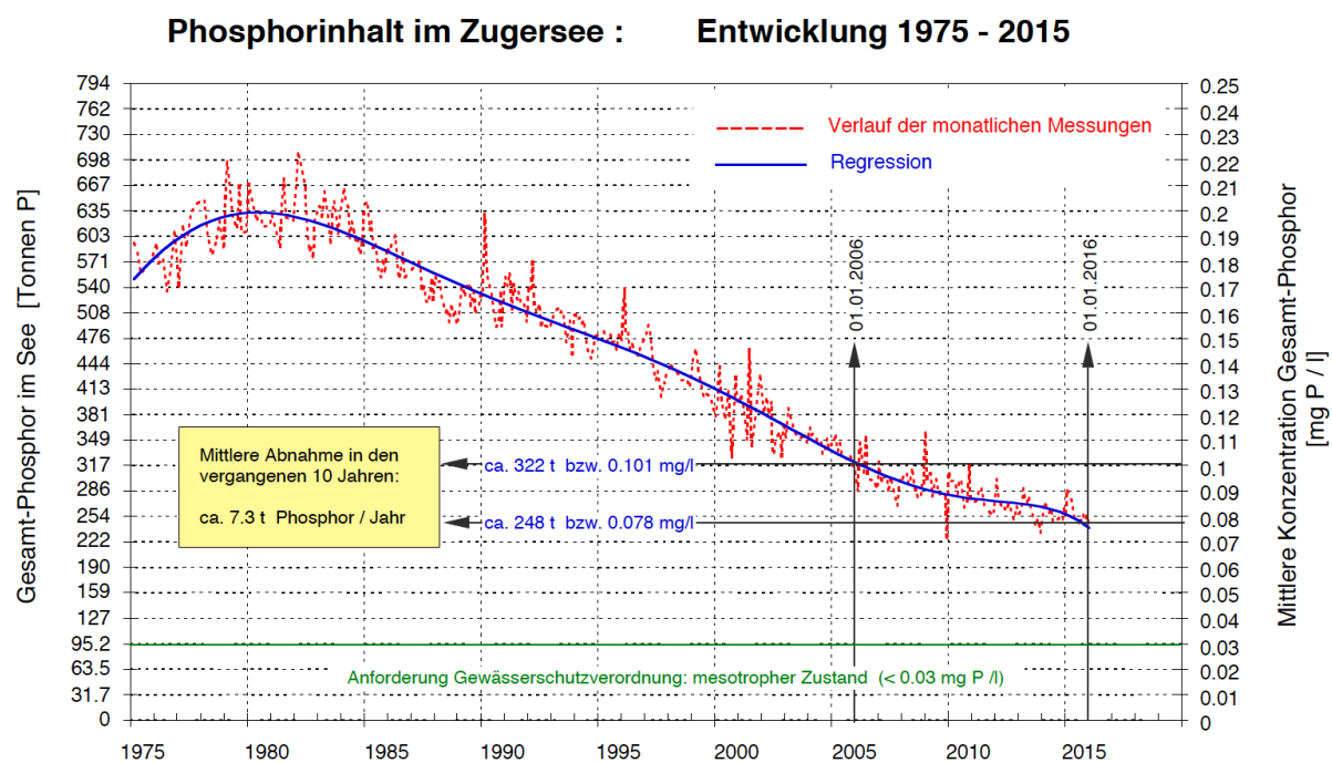
Figur A1: Zeitlicher Verlauf von Menge und mittlerer Konzentration von Gesamtphosphor im Zugersee von 1975 bis 2015. Quelle: AfU Zug.
