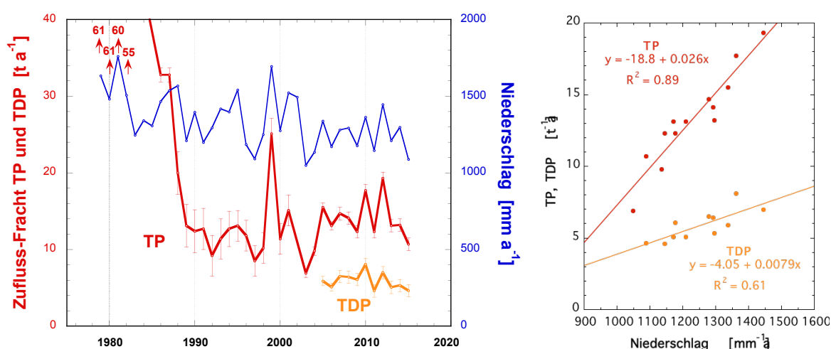
Figur 2: a) Korrelation der aus dem Zuflussmonitoring berechneten Frachten von TP und TDP mit dem jährlichen Niederschlag. Der Jahresniederschlag wurde als Mittel der Stationen Zugerberg, Lorzetobel und Cham berechnet. b) Linearer Zusammenhang zwischen Niederschlag und Fracht wurden aus den Zuflussdaten seit 2003 - 2015 (TP) bzw. 2005 - 2015 (TDP) berechnet.
