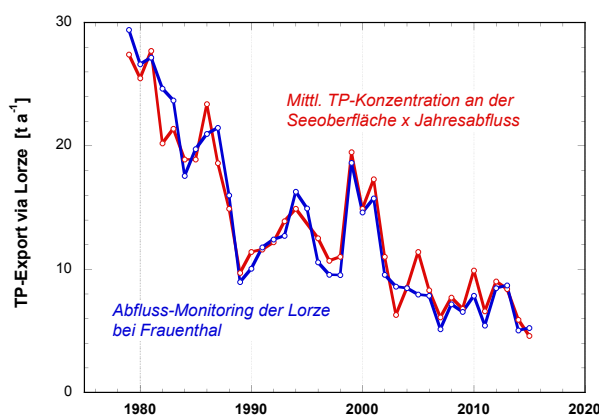
Figur 4: Vergleich verschiedener Berechnungsarten des P-Exports aus dem See. Rot: als Produkt von Jahresabfluss und gemittelter Oberflächenkonzentration des Sees. Blau: Monitoring der Lorze bei Frauenthal, Abzüglich des Zwischeneinzugsgebiets Cham-Frauenthal sowie ARA Schönaus.
