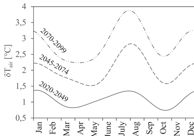
Figur A4: Saisonaler Verlauf der erwarteten Erwärmung der Atmosphäre gemäss CH2011 gegenüber heute (1980 – 2009) für das IPCC Entwicklungsszenario A1B für die Station Göttingen und drei künftige Zeiträume. Der Unterschied zwischen Sommer und Winter verstärkt sich in Zukunft.
