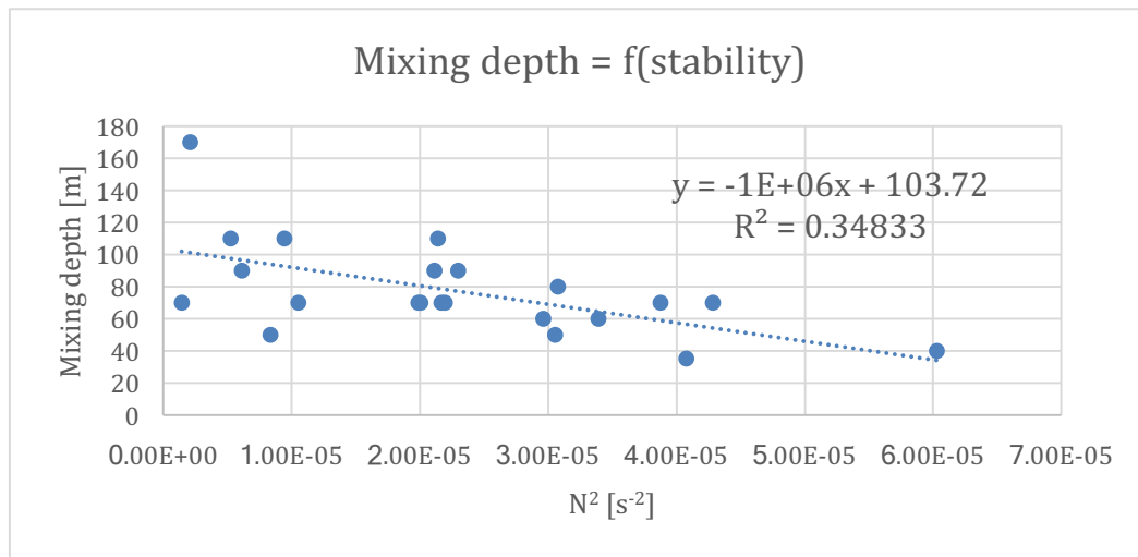
Figur A2: Maximale Mischungstiefe für die Zeitperiode seit Winter 1993/94 als Funktion der Stabilität der Wassersäule im November vor der winterlichen Abkühlung (Tabelle A2). Der Umstand, dass zwischen diesen beiden Grössen ein deutlicher Zusammenhang besteht, deutet darauf hin, dass auch die Abkühlung im Herbst (nicht nur die Temperaturen im Winter) einen starken Einfluss auf die Tiefenmischung hat.
