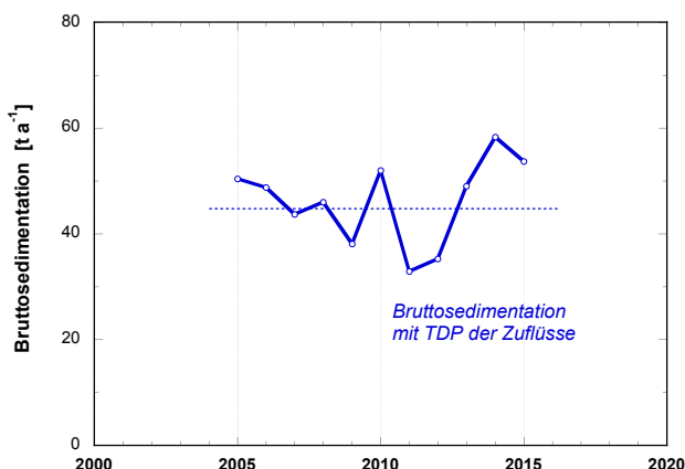
Figur 8: Bruttosedimentation von P (Netto-Export aus dem Epilimnion (25 m)) nach Gleichung 3 berechnet. Für die Zulauf-Fracht wurde das biologisch verfügbare, gesamt-gelöste P (TDP) verwendet.
