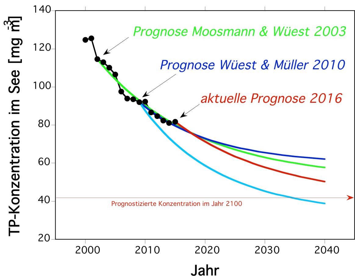
Figur 11: Messungen der Jahresmittel von TP im Zugersee (schwarze Punkte) und Prognosen. Im Jahr 2003 wurde die Prognose von Moosmann und Wüest verfasst (grün) und in 2010 die Prognose von Wüest und Müller (hell- und dunkelblau; unter Verwendung der NS aus dem P-Budget (hellblau) bzw. aus den Sedimentanalysen (dunkelblau)). Die rote Kurve ist die aktuelle Extrapolation aus dem vorliegenden Bericht. Im Jahr 2100 würde eine Konzentration von 42 \text{ mg m}^{-3} erreicht.
