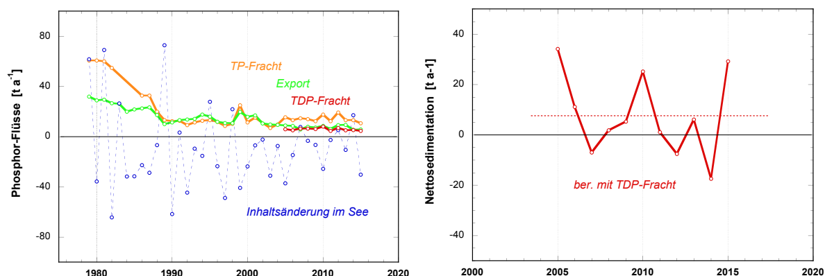
Figur 6: a) Jährliche Fracht von TP (orange) bzw. TDP (rot) aus den Zuflüssen, Export aus dem See (grün) und der Änderung des TP-Seeinhalts jeweils von Feb/März zu Feb/März des folgenden Jahres (blau), berechnet aus den im Zugersee erhobenen Monitoringdaten. b) Nettosedimentation berechnet aus dem Budget (Gleichung 2) unter Verwendung von TDP aus den Zuflüssen.
