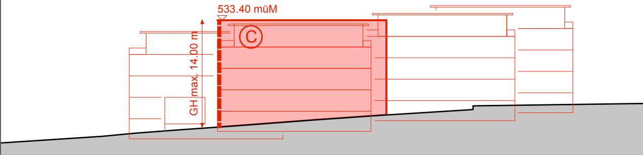
Schemaschnitt C–C
