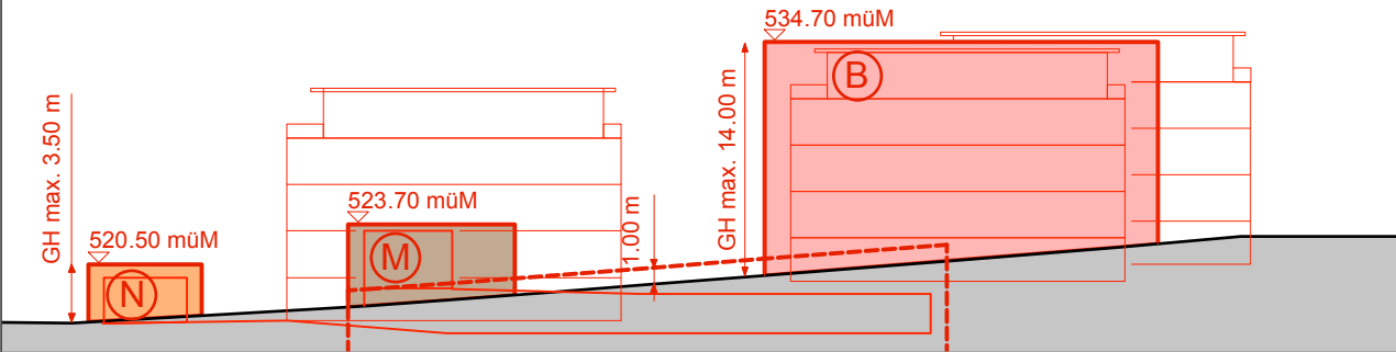
Schemaschnitt B–B
