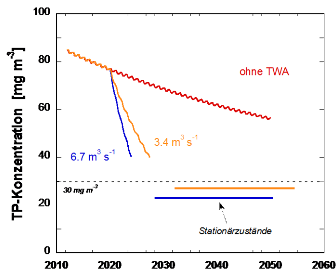
Figur 9: Konzentration von Gesamt-Phosphor (TP) nach der Winterzirkulation im Zugersee für zwei Szenarien der Tiefenwasserableitung in die Reuss bei unverändertem Abfluss der Lorze. Für den Beginn der Massnahmen wurde das Jahr 2020 angenommen. Die zeitliche Entwicklung bis zur Erreichung der Stationärzustände kann nicht verlässlich modelliert werden, weil sich der Austausch zwischen Epi- und Hypolimnion verändert.
