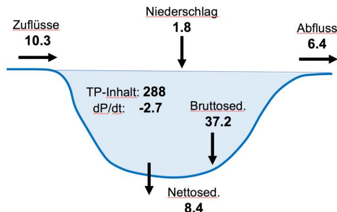
Figur 4. Aktuelle Phosphorbilanz des Zugersees. Zahlen sind in \text{tP a}^{-1} , gemäss Daten der Tabelle 2.
