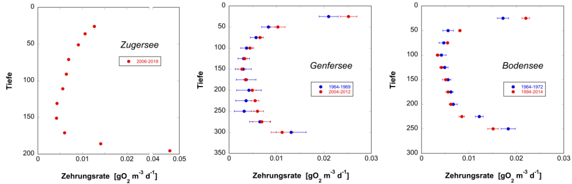
Figur 10: Sauerstoff-Volumenzehrung [ \text{g m}^{-3} \text{ d}^{-1} ] in der Wassersäule vom Zugersee, Genfersee und Bodensee während der Zeit der eutrophen Phase (blau, Genfersee 1964-1969; Bodensee 1964-1972) und seit der Re-Oligotrophierung (rot, Genfersee 2004-2012; Bodensee 1994-2014). (Aus Schwefel et al., in Vorbereitung). Die Zehrung im Tiefenwasser des Zugersees beruht vor allem auf der grossen Freisetzung von \text{CH}_4 und \text{NH}_4^+ .
