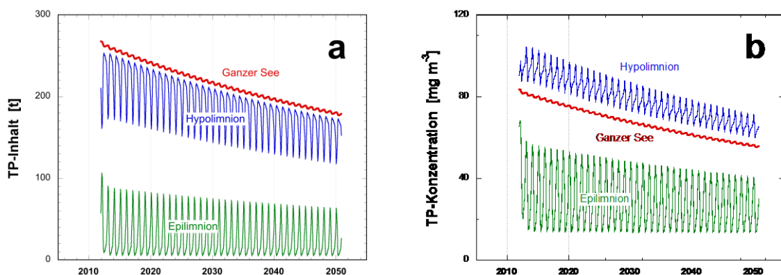
Figur 5: Künftiger zeitlicher Verlauf von TP-Inhalt (a) und volumen-gewichteter mittlerer Konzentration (b) bis 2050 für den gesamten See (rot), das Epilimnion (grün) und das Hypolimnion (blau). Das 2-Box-Modell berücksichtigt die im jahreszeitlichen Rhythmus sich ändernde Produktionstiefe (bestimmt aus der Lage des TP-Konzentrationsgradienten; Tabelle 3) und die mittleren monatlichen Wasser- und TDP-Frachten.
