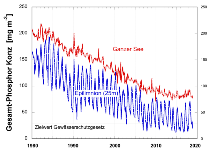
Figur 2. Volumengewichtete mittlere TP-Konzentrationen für die gesamte Wassersäule (rot) und das Epilimnion (blau) seit 1980. Die schwarze Linie bezeichnet den Zielwert von 30 \text{ mg m}^{-3} ( 96 \text{ tP} ).
