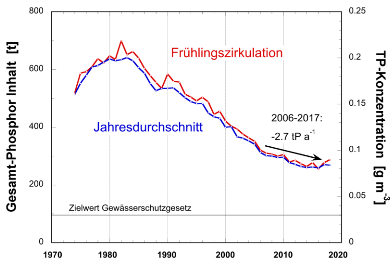
Figur 1. Verlauf der Menge und Konzentration von Gesamtphosphor (TP) im Zugersee während der Frühlingszirkulation (rot, Maximum der Monate Februar bis April) und als Jahresmittelwerte (blau). Die Abnahmerate wurde berechnet als mittlere Differenz der Zirkulationswerte zwischen 2006 und 2017 ( -2.7 \text{ tP a}^{-1} ). Die schwarze Linie bezeichnet den Zielwert von 30 \text{ mg m}^{-3} ( 96 \text{ tP} ) für mittlere Produktion.
