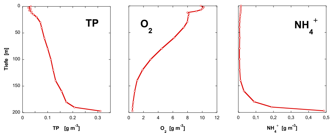
Figur 3: Gemittelte vertikale Konzentrationsprofile von TP, O_2 und NH_4^+ in der Wassersäule des Zugersees. Mittelwerte von monatlichen Messungen der Jahre 2006 bis 2018.
