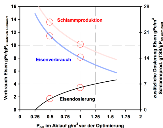
Figur 12: Anstieg des spezifischen Verbrauchs an Fällmittel und der Fällschlamm-Produktion in Abhängigkeit des zusätzlich gefällten gelösten Anteils im Ablauf der Kläranlagen (Beispielrechnung für eine gelöste P-Konzentration von 4.9 \text{ g/m}^3 , Angaben \pm 15\text{-}20\% ). Aus Böhler und Siegrist (2008, S. 75).
