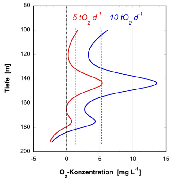
Figur 11: Konzentrationsprofile von Sauerstoff im Zugersee unterhalb von 100 m Wassertiefe bis zum Grund, modelliert für Einträge von 5 \text{ tO}_2 \text{ d}^{-1} (rot) und 10 \text{ tO}_2 \text{ d}^{-1} (blau). Für diese Berechnungen wurde die turbulente Mischung, die auch bei der permanenten Dichteschichtung immer noch in geringem Umfang vorhanden ist, nicht berücksichtigt. Durch die vertikale Diffusion würden die Maxima (bis 14 \text{ mgO}_2 \text{ L}^{-1} ) und Minima (bis -2.5 \text{ mgO}_2 \text{ L}^{-1} ) abgeflacht.
