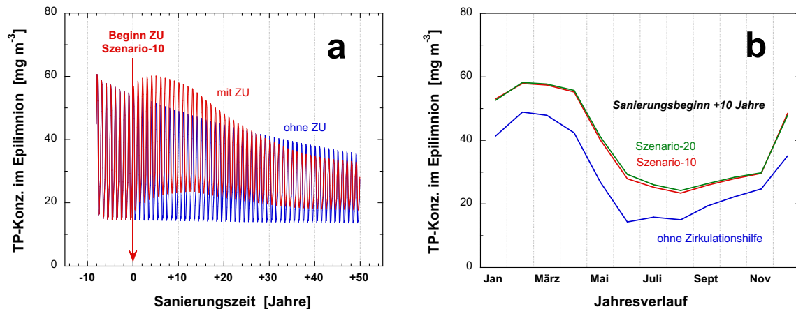
Figur 3: Auswirkungen der ZU auf die P-Konzentration bei Absenkung der Diffusoren um 10 m pro Jahr. (Konstante Eintragsfracht von 12.1 \text{ t P a}^{-1} ).
