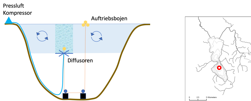
Figur 1: Links: Prinzip der Positionierung der Diffusoren. Die Mischungstiefe wird jeden Winter um 10 bis 20 m abgesenkt, bis die maximale Tiefe erreicht ist. Rechts: Lage der Diffusoren im Bereich der tiefsten Stelle im Südbecken.
