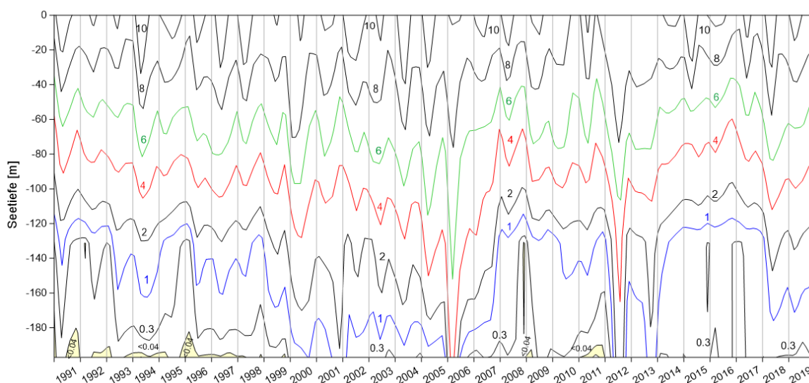
Figur 6: Sauerstoffverteilung im Zugersee von 1991 bis 2019 in \text{mg L}^{-1} (AFU Zug).
