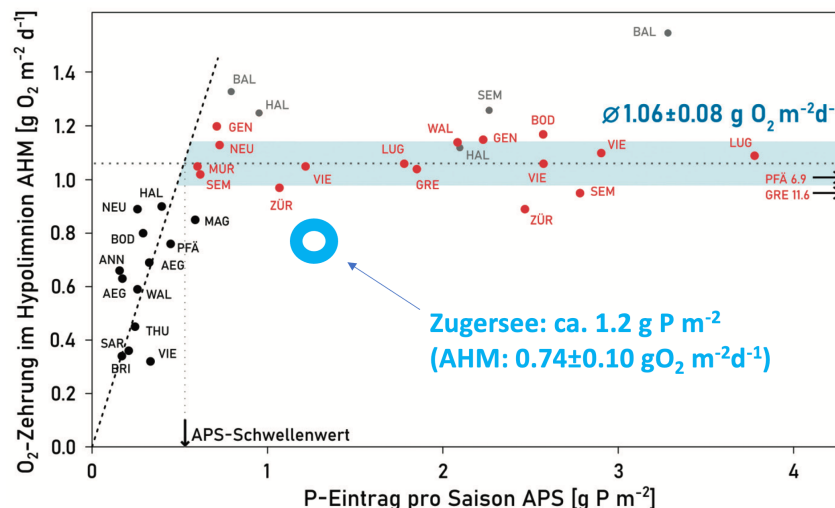
Figur 5: Abhängigkeit der Sauerstoffzehrung im Tiefenwasser vom für das Algenwachstum zur Verfügung stehenden Phosphor. Durch den Betrieb der ZU wird die AHM bis \sim 1.06 \text{ g O}_2 \text{ m}^{-2} \text{ d}^{-1} zunehmen. Wenn die APS durch die Wirkung der see-internen wie -externen Massnahmen unter die Schwelle von 0.6 \text{ g P m}^{-2} sinkt, wird auch die AHM abnehmen. (aus Kiefer et al., 2021).
