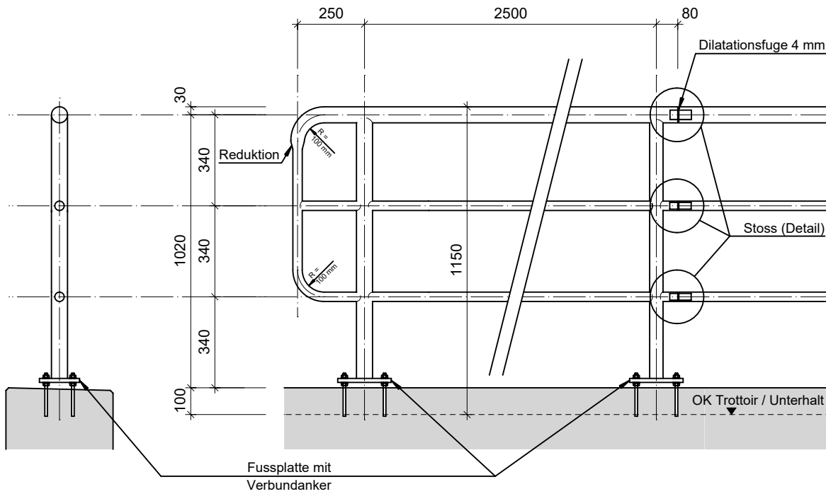
Schnitt 1:20
